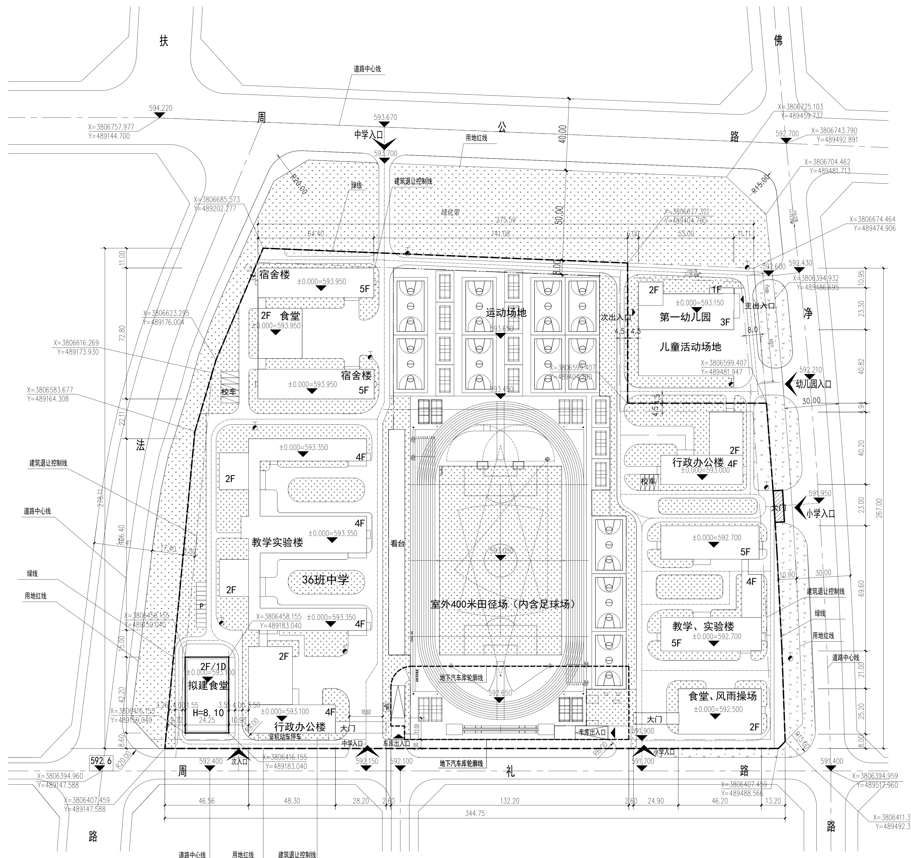
总平面图 1:1000
